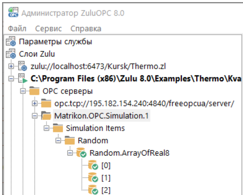
Рисунок 3.12. Значения из массива, отображаемые как подтеги OPC
