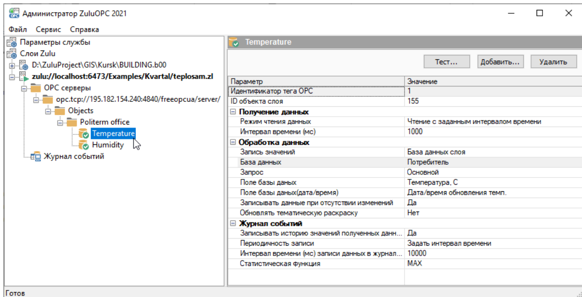
Рисунок 3.10. Параметры OPC-тега
