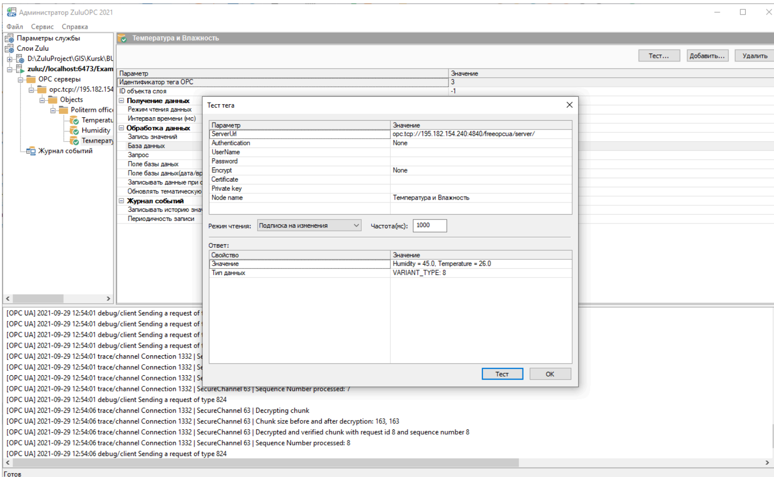
Рисунок 3.16. Журнал сообщений Администратор ZuluOPC
