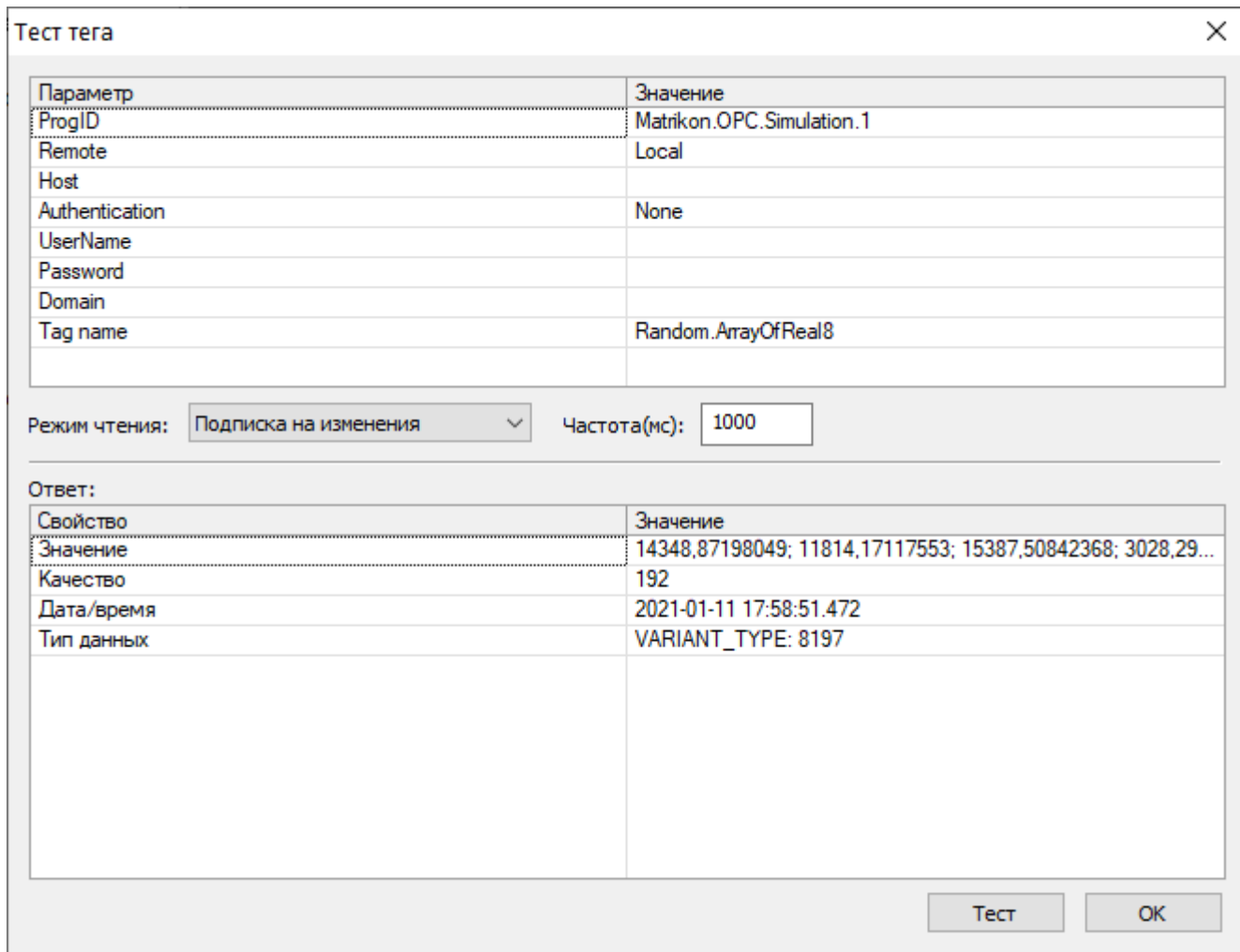
Рисунок 3.14. Значения из массива, отображаемые как подтеги OPC
