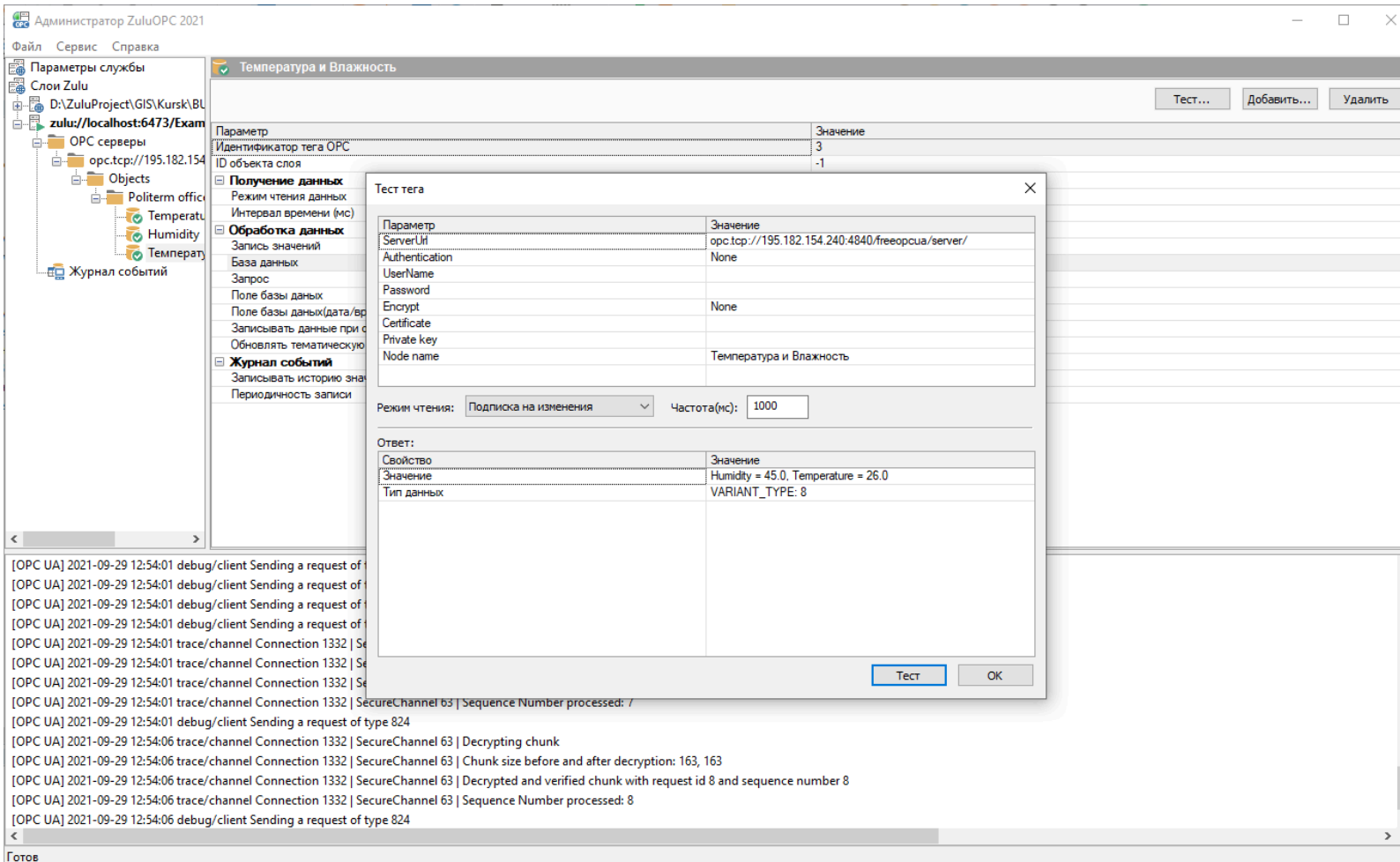
Рисунок 3.11. Тестирование настроек OPC-тега
